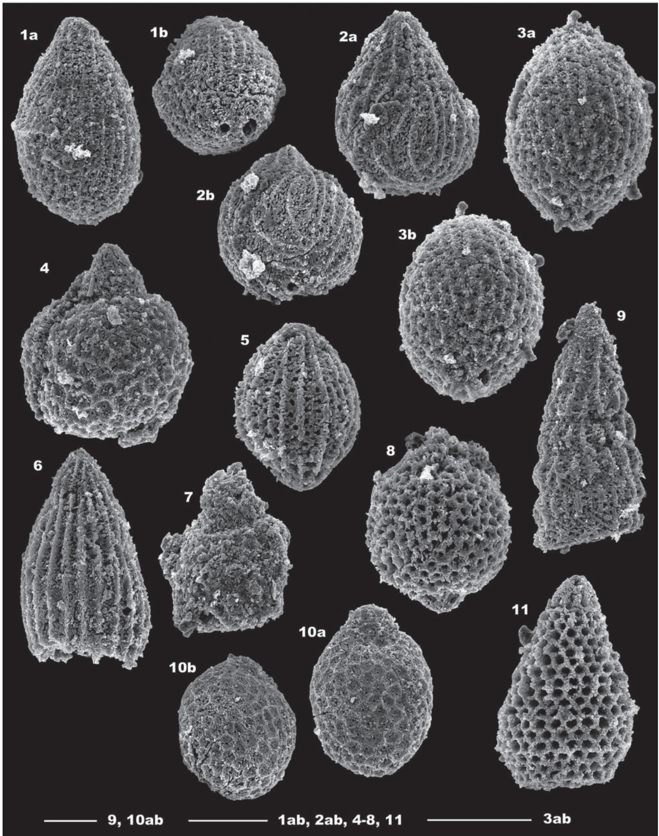
図版 1 小沢層のチャート礫から得られたジュラ紀放射虫化石 (試料 1-48) の電子顕微鏡写真。スケールは 0.05 mm.
