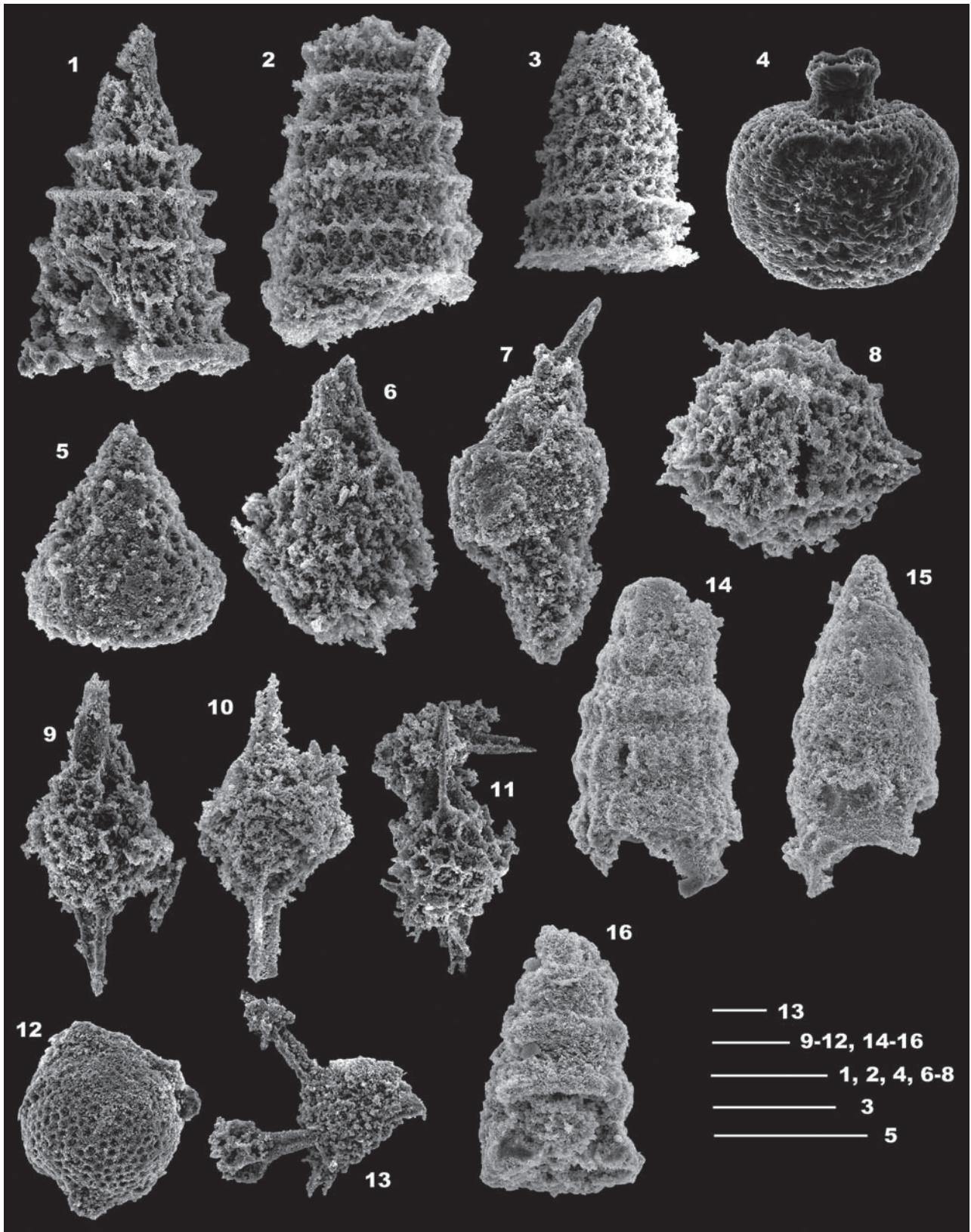
図版 2 小沢層のチャート礫から得られたジュラ紀放射散虫化石 (試料 1-79) とジュラ紀～白亜紀放射散虫化石 (試料 03022806-12) . スケールは 0.05 mm.
