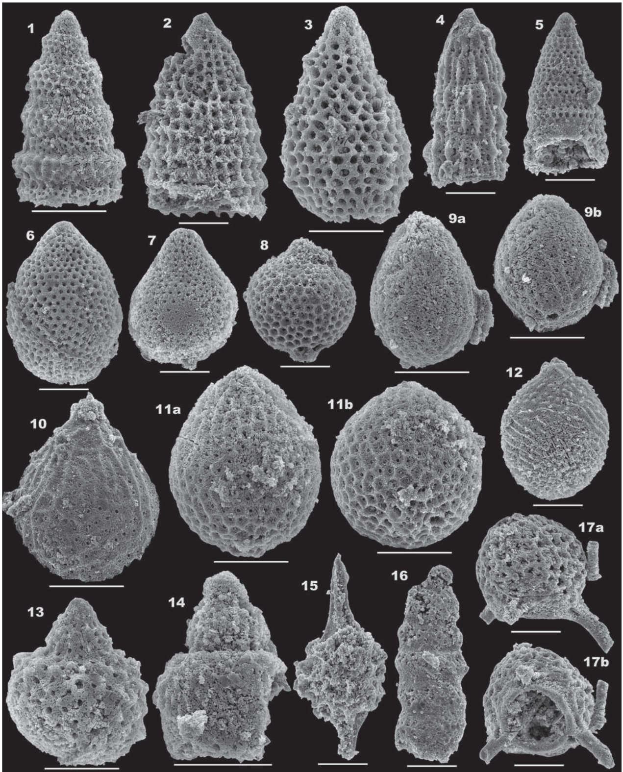
図版4 神沢層の泥質チャート礫から得られたジュラ紀放射虫化石(試料 98032501-17), およびチャート礫から得られた三畳紀放射虫化石(試料 98032501-16)の電子顕微鏡写真. スケールは 0.05 mm.
